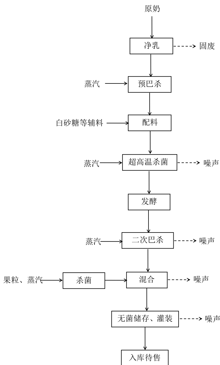
图3 笑脸杯生产工艺及产污环节示意图
