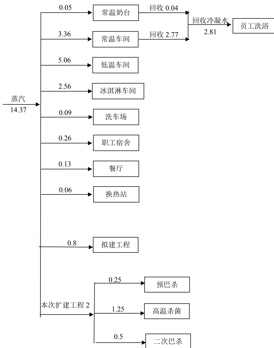
图 1 扩建工程完成后全厂蒸汽平衡图 单位：t/h
