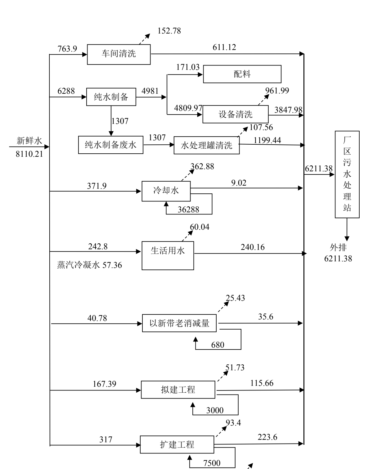
图 6 扩建工程完成后全厂水平衡图 代表散失量 单位：
