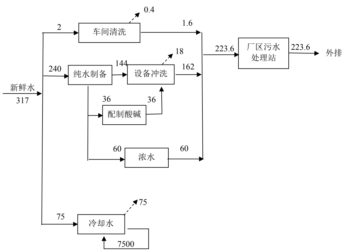
图 5 扩建工程水平衡图 代表散失量 单位：m 3 /d
