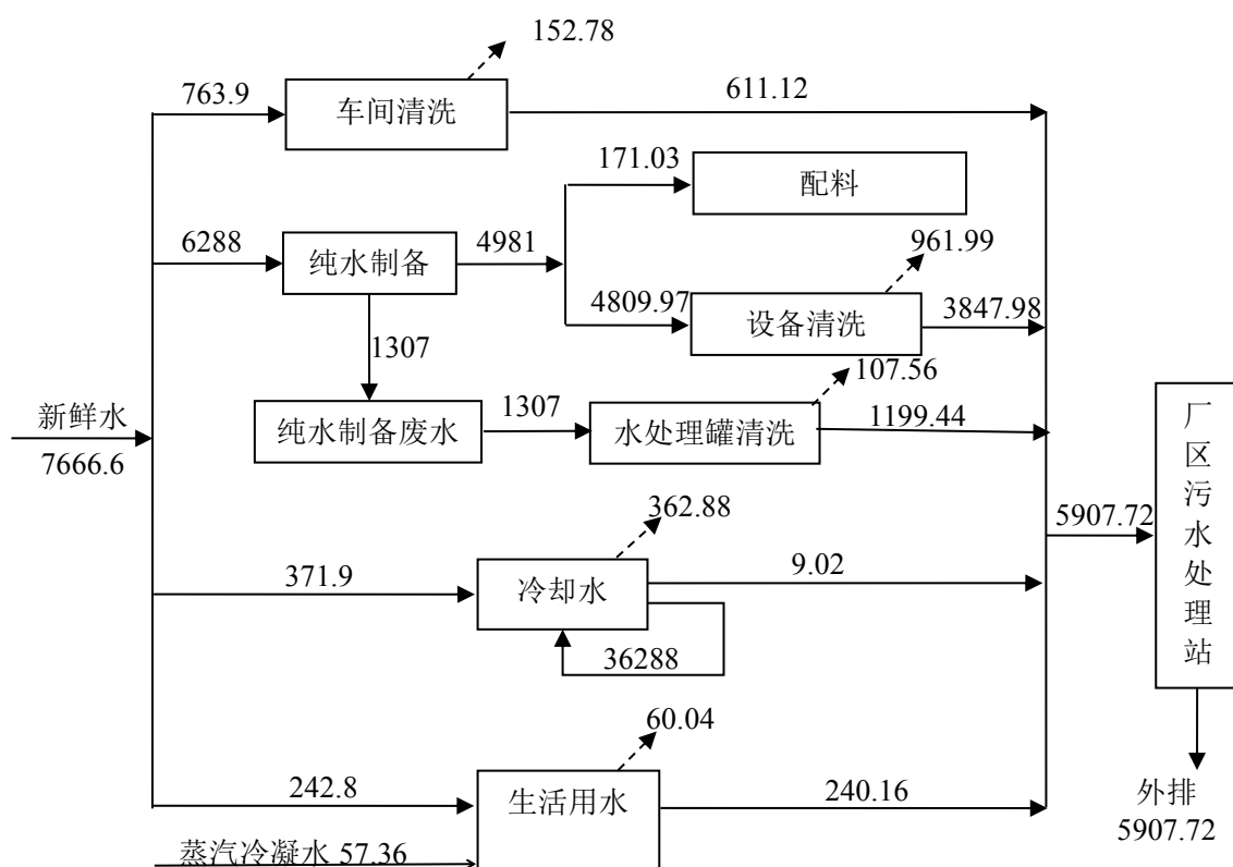
图 6 现有工程水平衡图 代表散失量 单位: \text{m}^3/\text{d}
