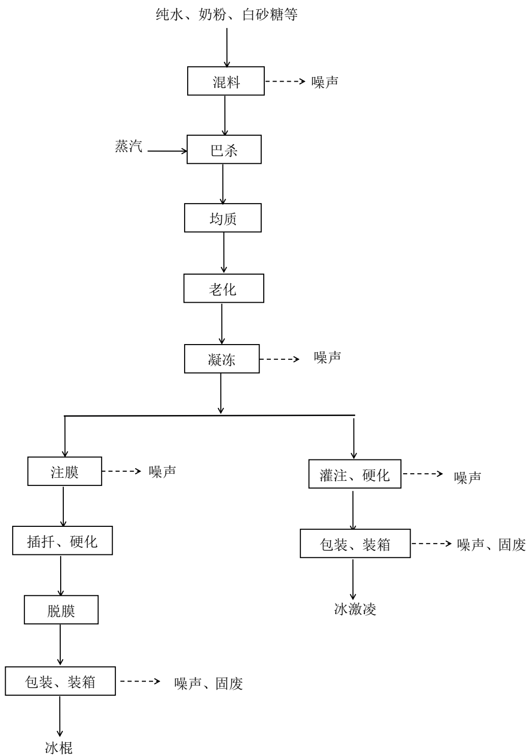
图 4 生产工艺及产污环节示意图
