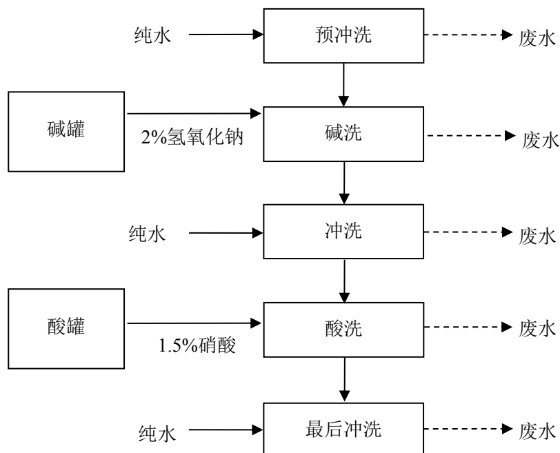
图 5 CIP 清洗工艺及产污环节流程图
