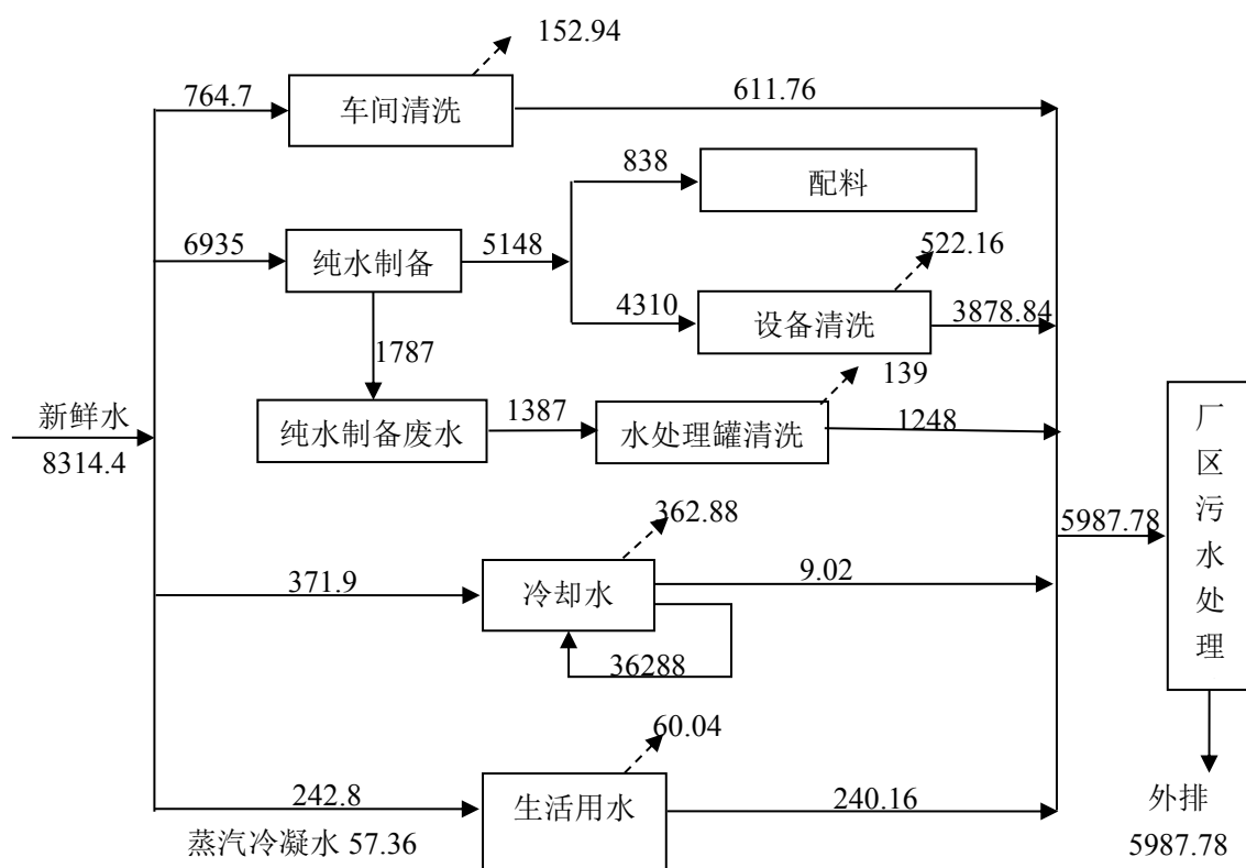
图1 现有工程水平衡图 代表散失量 单位: m³/d
