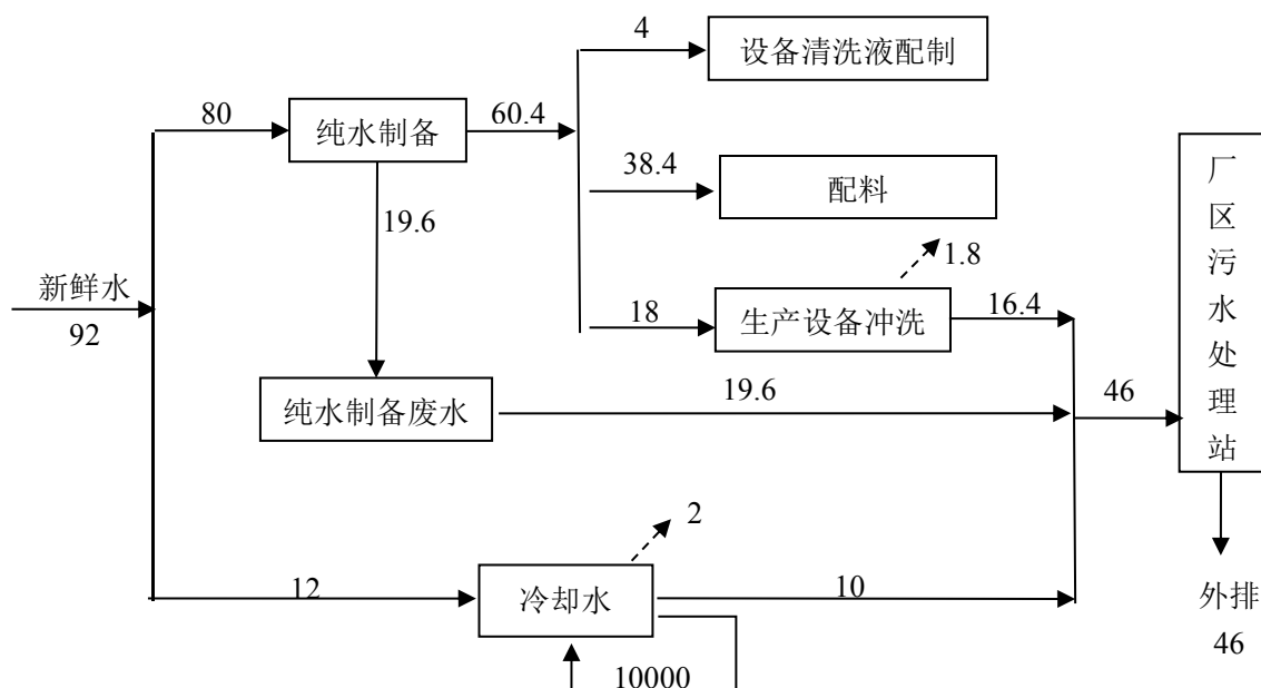
图 7 本次工程水平衡图 代表散失量 单位：m 3 /d
