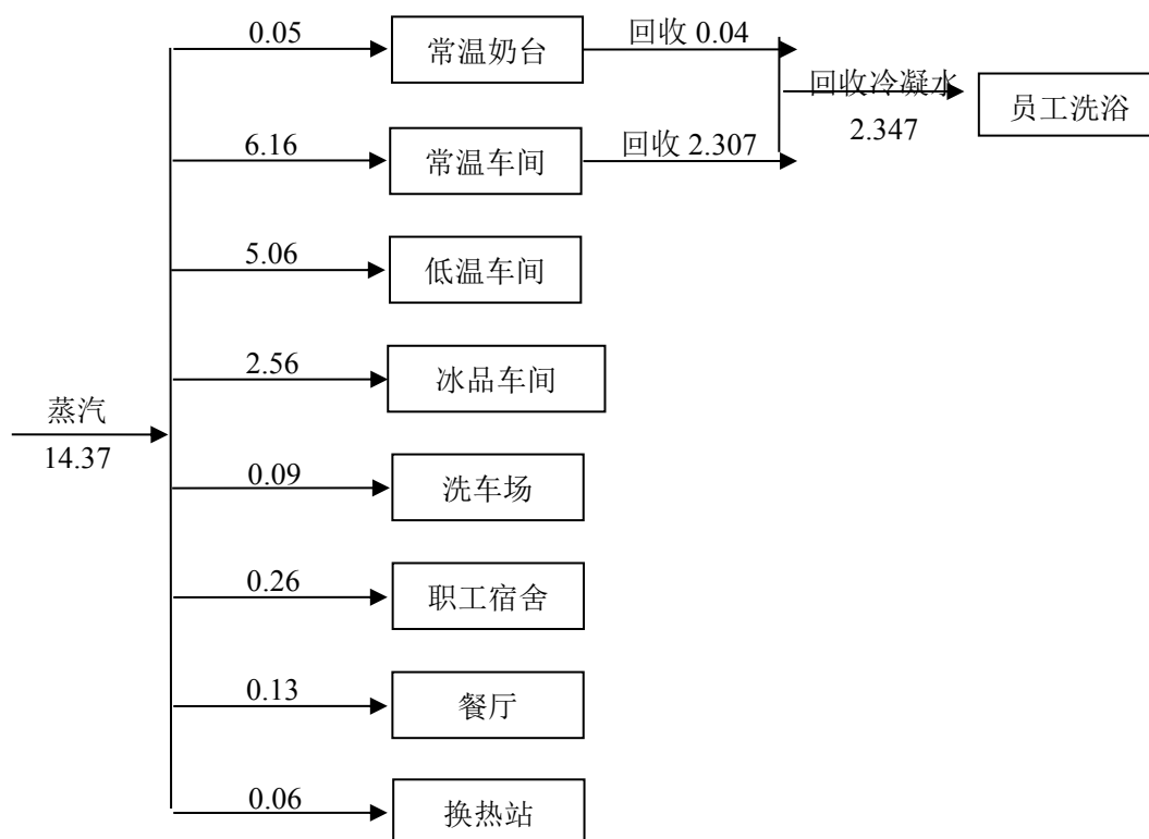
图2 厂区现有工程蒸汽平衡图 单位：t/h
